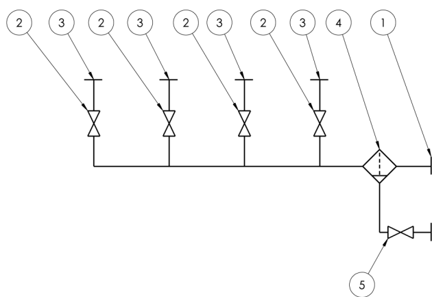
Рис. 3.2 Пневматическая схема КС-4-Т
