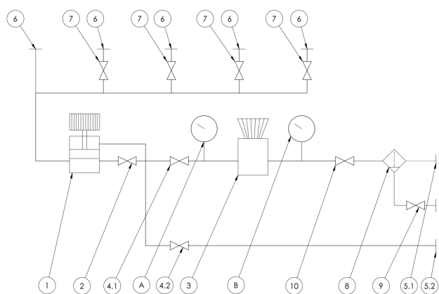
Рис. 1. Пневматическая схема КС-55-Т
