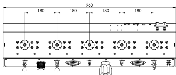
Рис. 1. Габариты КС-55 и КС-55-Т
